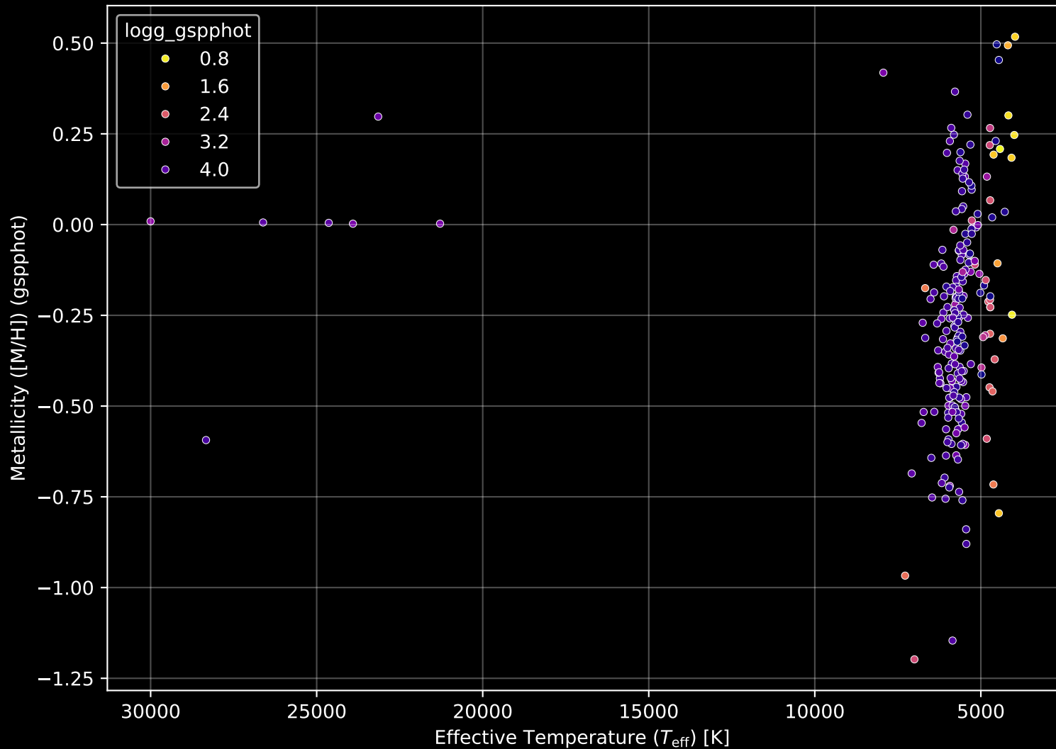
GALAH DR4 Field: [727] Stellar Population Parameters (n= 231)
