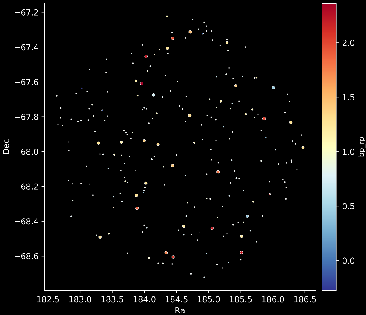
GALAH DR4 Field: [727] Stars: 231
